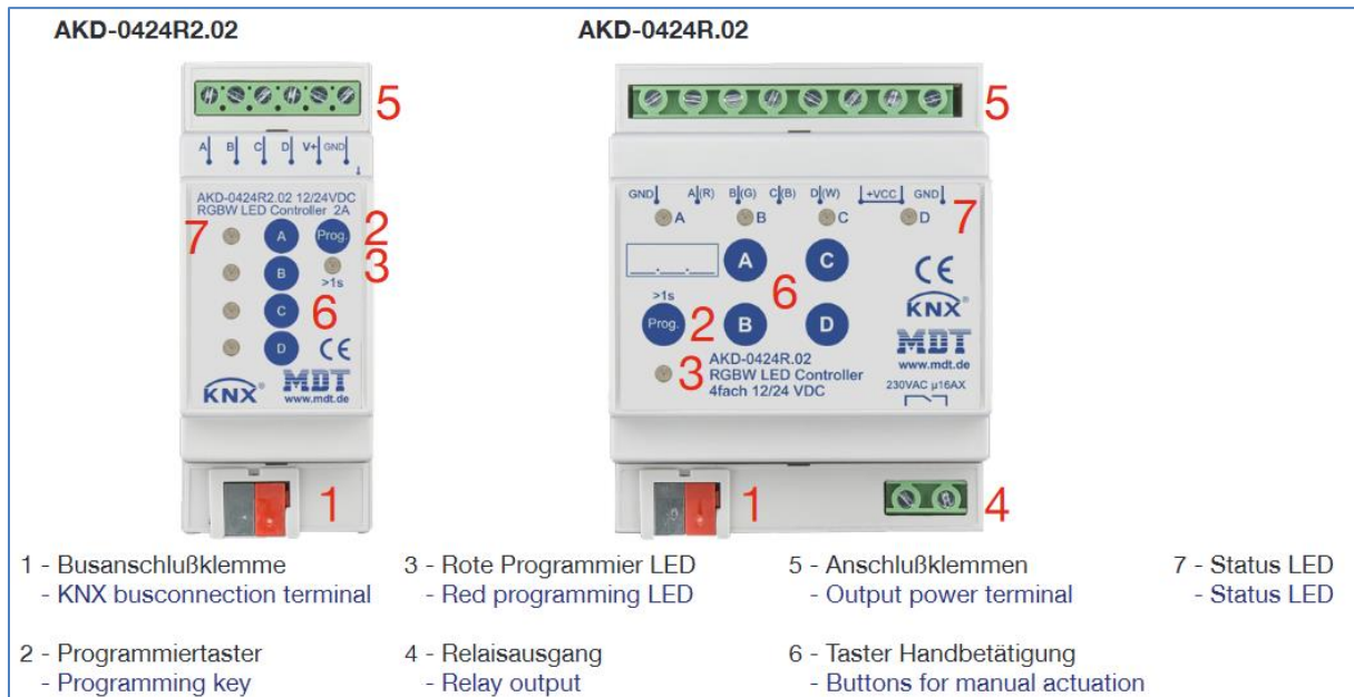
Abbildung 1: Aufbau Hardwaremodul REG
