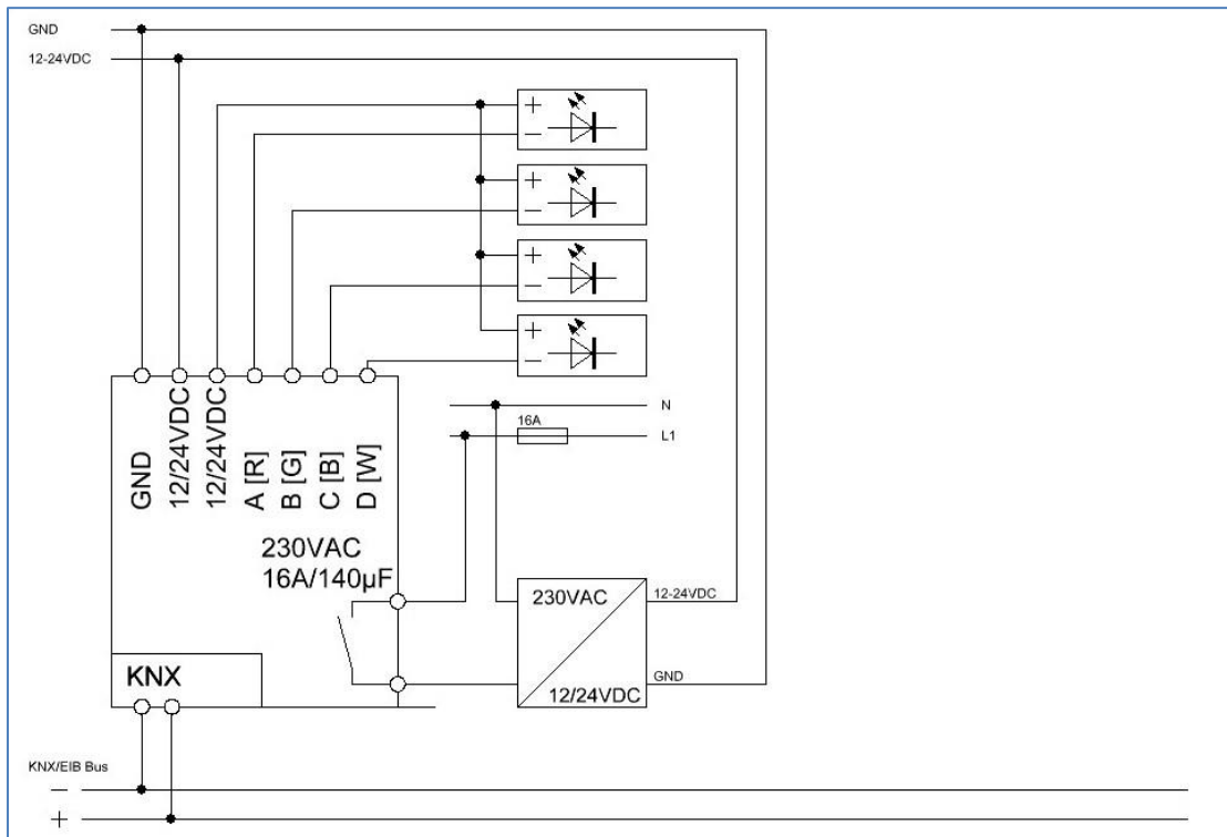
Abbildung 3: Exemplarisches Anschlussschema, hier AKD-0424V.02
