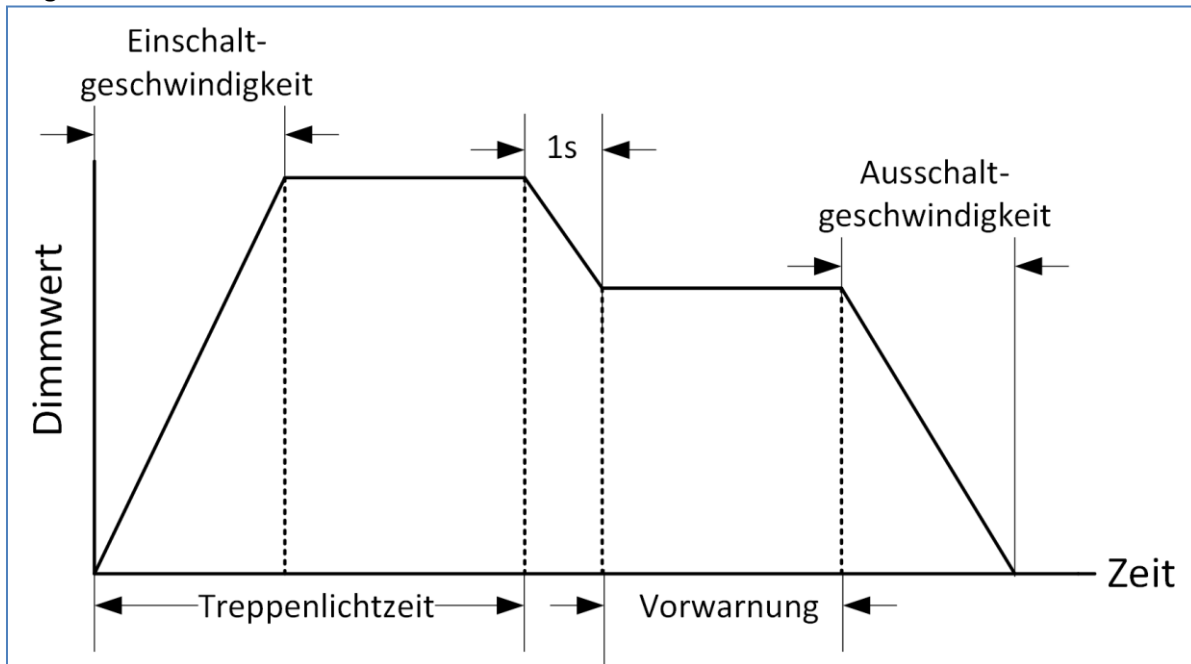
Abbildung 14: Ablaufdiagramm – Treppenlicht mit Dimmzeiten
