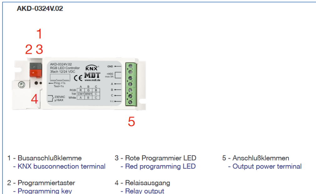
Abbildung 2: Aufbau Hardwaremodul Aufputz Geräte
