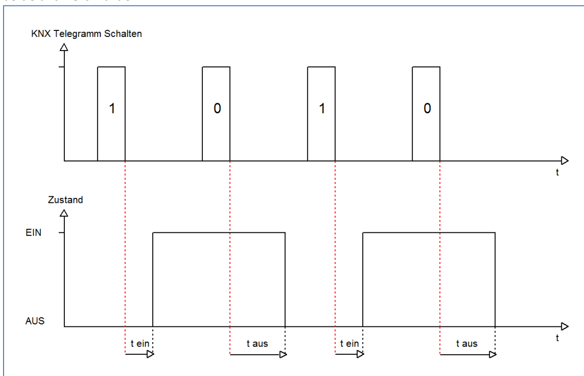
Abbildung 11: Funktionsdiagramm – Ein-/Ausschaltverzögerung
